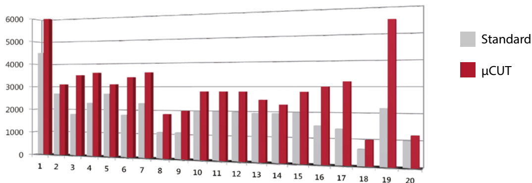
Versuchsreihe Verzahnung Abwälzfräser, verschiedene Werkzeuge
